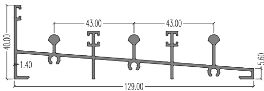
5083 (Bottom Outer) LW : 1.361 kg/m AP : 669.07 mm
