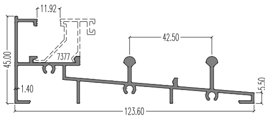
5094 (Bottom Outer) LW : 1.263 kg/m AP : 598.90 mm
