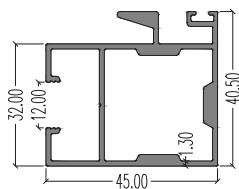
7969 (Interlock) LW : 0.940 kg/m AP : 295.67 mm Ixx : 6.771 cm 4 Iyy : 7.108 cm 4
