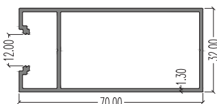
5010 (Side Inner) LW : 0.783 kg/m AP : 276.13 mm
