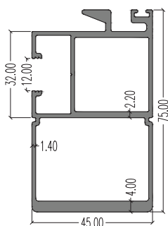
7934 (Interlock) LW : 1.705 kg/m AP : 362.45 mm Ixx : 44.68 cm 4 Iyy : 14.60 cm 4
