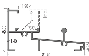
7376 (Bottom Outer) LW : 0.916 kg/m AP : 453.80 mm
