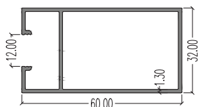
7967 (Side Inner) LW : 0.707 kg/m AP : 254.89 mm
