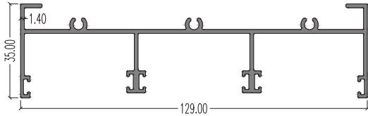
5084 (Top & Side Outer) LW : 1.199 kg/m AP : 628.78 mm
