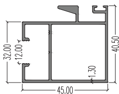
7968 (Interlock) LW : 0.769 kg/m AP : 296.11 mm Ixx : 5.911 cm 4 Iyy : 6.241 cm 4
