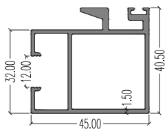
7365 (Interlock) LW : 0.865 kg/m AP : 291.61 mm Ixx : 6.577 cm 4 Iyy : 6.850 cm 4
