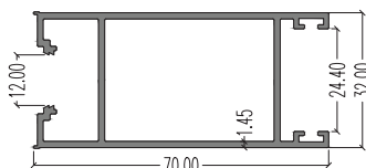
7935 (Intermediate) LW : 0.904 kg/m AP : 330.66 mm
