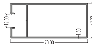
7979 (Side Inner) LW : 0.776 kg/m AP : 274.48 mm
