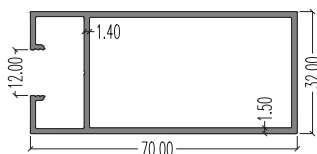
7366 (Side Inner) LW : 0.859 kg/m AP : 274.34 mm
