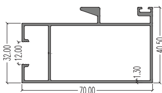
7980 (Interlock) LW : 0.957 kg/m AP : 346.63 mm Ixx : 7.689 cm 4 Iyy : 19.52 cm 4
