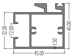
7369 (Interlock) LW : 0.955 kg/m AP : 290.06 mm Ixx : 6.725 cm 4 Iyy : 7.448 cm 4
