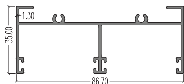
7049 (Top & Side Outer) LW : 0.858 kg/m AP : 474.48 mm
