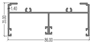
7379 (Top & Side Outer) LW : 0.860 kg/m AP : 468.41 mm
