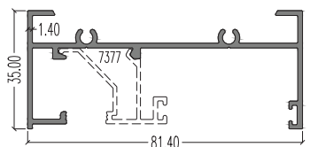
7373 (Top & Side Outer) LW : 0.789 kg/m AP : 408.15 mm
