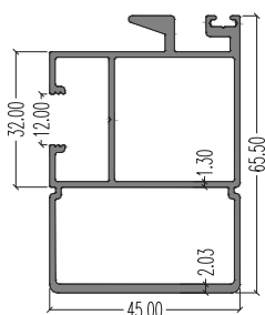
5125 (Interlock) LW : 1.230 kg/m AP : 345.61 mm Ixx : 23.47 cm 4 Iyy : 11.12 cm 4
