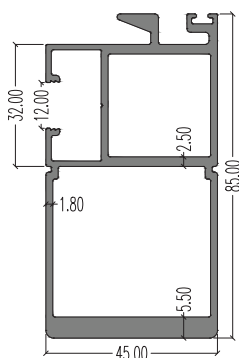
5155 (Interlock) LW : 2.144 kg/m AP : 381.75 mm Ixx : 71.68 cm 4 Iyy : 18.93 cm 4
