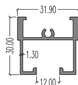
7375 (Top Inner) LW : 0.534 kg/m AP : 237.44 mm
