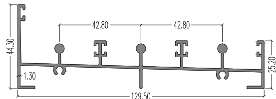
7040 (Bottom Outer) LW : 1.352 kg/m AP : 688.85 mm
