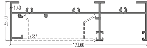
7372 (Top & Side Outer) LW : 1.203 kg/m AP : 628.89 mm
