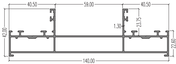
46932 (Outer) LW : 1.671 kg/m AP : 550.33 mm
