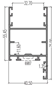
46962 (Inner) LW : 1.004 kg/m AP : 394.21 mm
