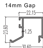
6996 (Beading) LW : 0.286 kg/m AP : 168.80 mm
