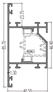
46964 (Transom) LW : 1.071 kg/m AP : 398.79 mm Ixx : 18.88 cm 4 Iyy : 8.846 cm 4
