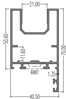
46961 (Inner) LW : 1.035 kg/m AP : 323.13 mm
