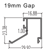
46902 (Beading) LW : 0.224 kg/m AP : 162.69 mm
