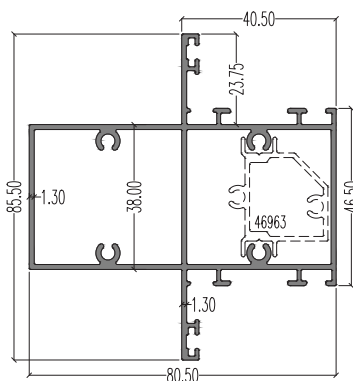
6977 (Mullion) LW : 1.495 kg/m AP : 451.00 mm Ixx : 22.17 cm 4 Iyy : 31.95 cm 4
