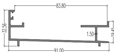
45393 (Subsill) LW : 0.744 kg/m AP : 376.55 mm
