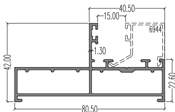
46928 (Outer) LW : 0.978 kg/m AP : 322.37 mm
