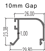
6986 (Beading) LW : 0.233 kg/m AP : 163.56 mm
