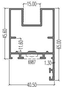
46930 (Inner) LW : 0.946 kg/m AP : 306.18 mm
