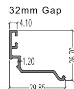
46965 (Beading) LW : 0.206 kg/m AP : 126.56 mm
