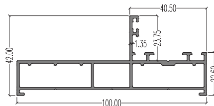
46960 (Outer) LW : 1.193 kg/m AP : 362.08 mm
