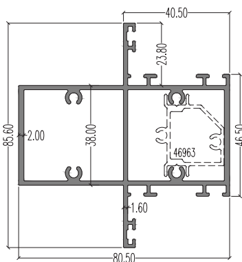
46900 (Mullion) LW : 1.829 kg/m AP : 454.30 mm Ixx : 25.38 cm 4 Iyy : 41.89 cm 4
