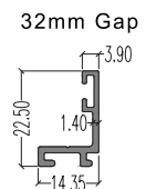
6218 (Beading) LW : 0.179 kg/m AP : 101.90 mm
