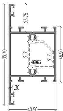
46929 (Mullion) LW : 1.028 kg/m AP : 377.38 mm Ixx : 18.50 cm 4 Iyy : 8.757 cm 4
