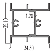
6976 (Bracket) LW : 0.553 kg/m AP : 214.74 mm Ixx : 2.163 cm 4 Iyy : 2.349 cm 4 (For 46929, 6977 & 14296)
