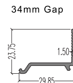
46910 (Beading) LW : 0.213 kg/m AP : 108.69 mm
