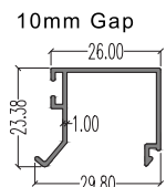
6985 (Beading) LW : 0.231 kg/m AP : 169.79 mm
