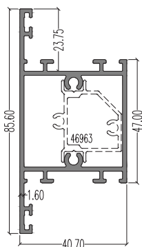
6993 (Mullion) LW : 1.211 kg/m AP : 375.44 mm Ixx : 21.05 cm 4 Iyy : 10.36 cm 4
