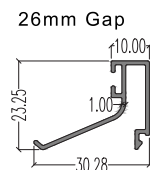
6997 (Beading) LW : 0.219 kg/m AP : 159.37 mm
