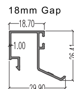
46917 (Beading) LW : 0.235 kg/m AP : 171.92 mm
