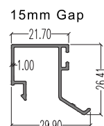
46918 (Beading) LW : 0.236 kg/m AP : 172.01 mm
