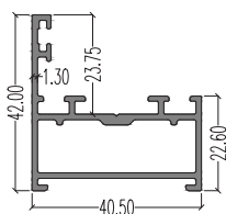
46927 (Outer) LW : 0.649 kg/m AP : 241.29 mm
