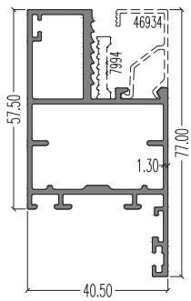
46933 (Inner) LW : 1.136 kg/m AP : 324.59 mm
