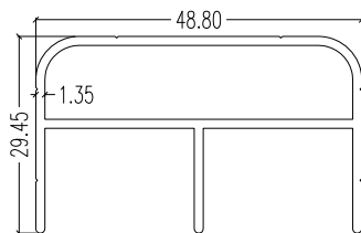
8730 LW : 0.619 kg/m AP : 213.22 mm
