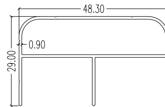
9888 LW : 0.393 kg/m AP : 211.90 mm
