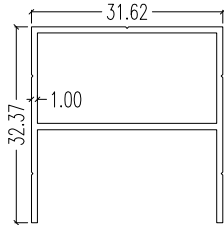
9831 LW : 0.340 kg/m AP : 159.76 mm
