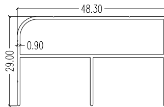
9830 LW : 0.401 kg/m AP : 214.57 mm
