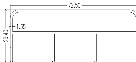
8727 LW : 0.867 kg/m AP : 292.98 mm
