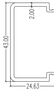
12643 LW : 0.477 kg/m AP : 187.66 mm
