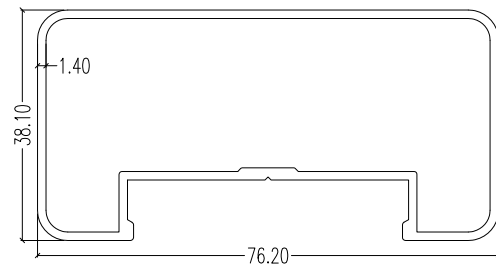
9613 LW : 0.926 kg/m AP : 243.05 mm
