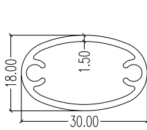
9609 LW : 0.349 kg/m AP : 77.92 mm
