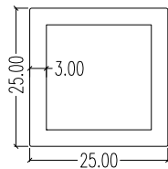
2726 LW : 0.716 kg/m AP : 99.48 mm
