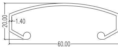
9611 LW : 0.428 kg/m AP : 210.35 mm
