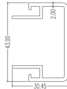
12642 LW : 0.624 kg/m AP : 257.65 mm
