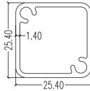
9610 LW : 0.396 kg/m AP : 95.56 mm
